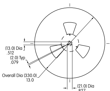
Reel Dimensions
