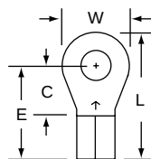
MU10-8R Stud Size 8 Wire Range 12-10
