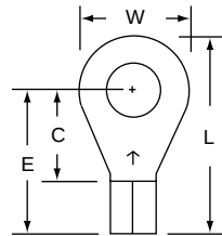
MU10-14R/S Stud Size 1/4 Wire Range 12-10
