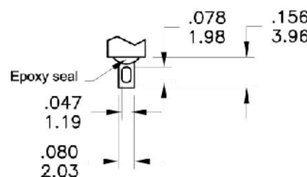
SOLDER LUG
