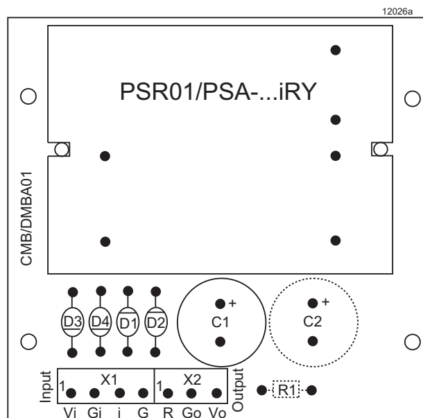
Fig. 13 C/DMBA01- .. PCB layout
