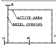
BEZEL/DISPLAY POSITION
