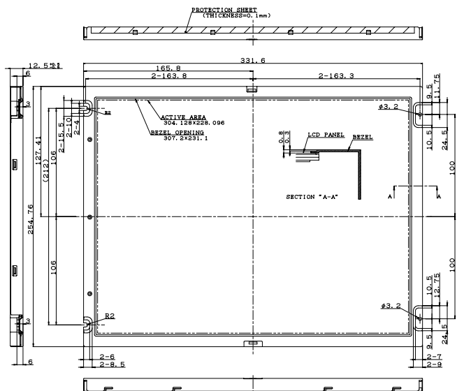
BEZEL/DISPLAY POSITION
