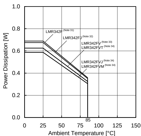
(d) LMR342xxx
