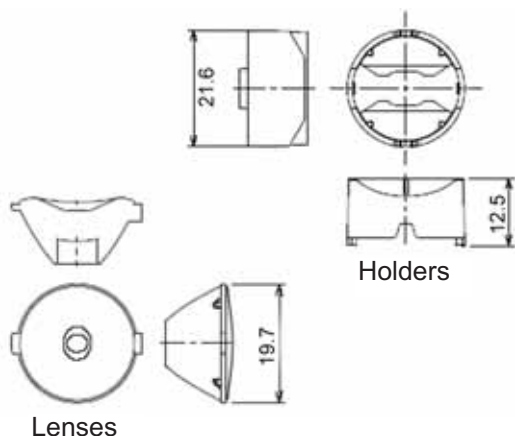
Lenses
