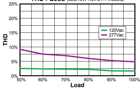
THD / Load (LED40W Rev E1.1 models)
