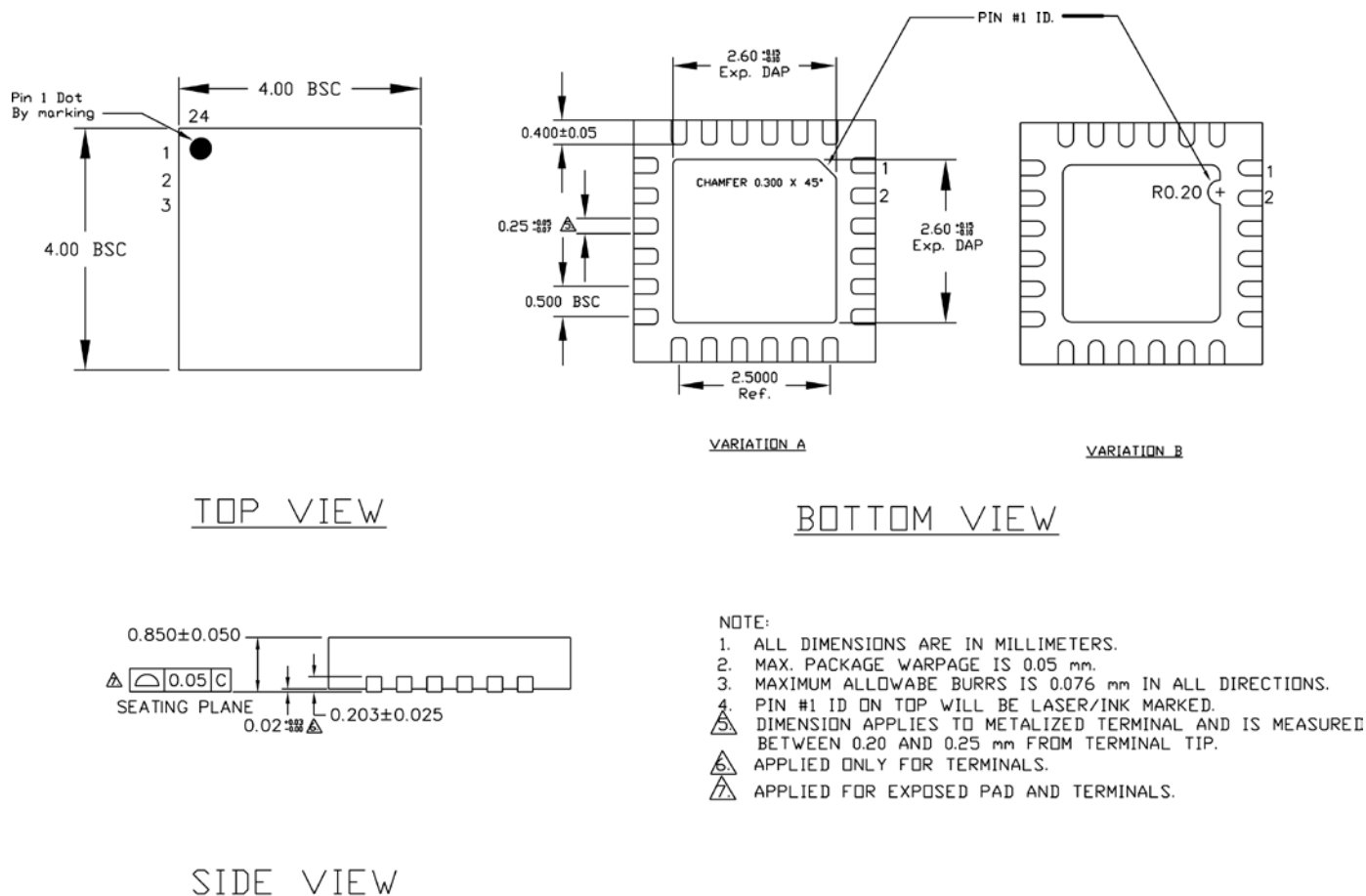
24-Pin QFN
