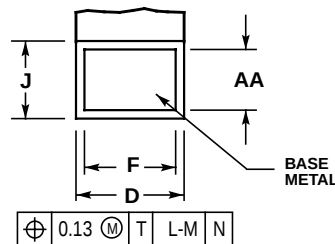
VIEW Y
