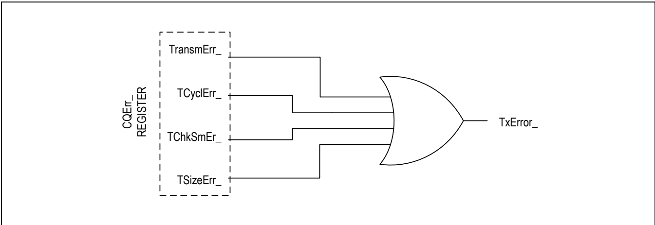
Figure 17. TxError_ Triggers
