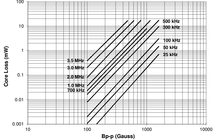
MPIA4012V2-2R2-R
