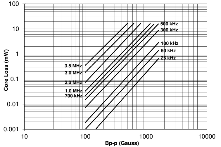
MPIA4012V2-1R0-R
