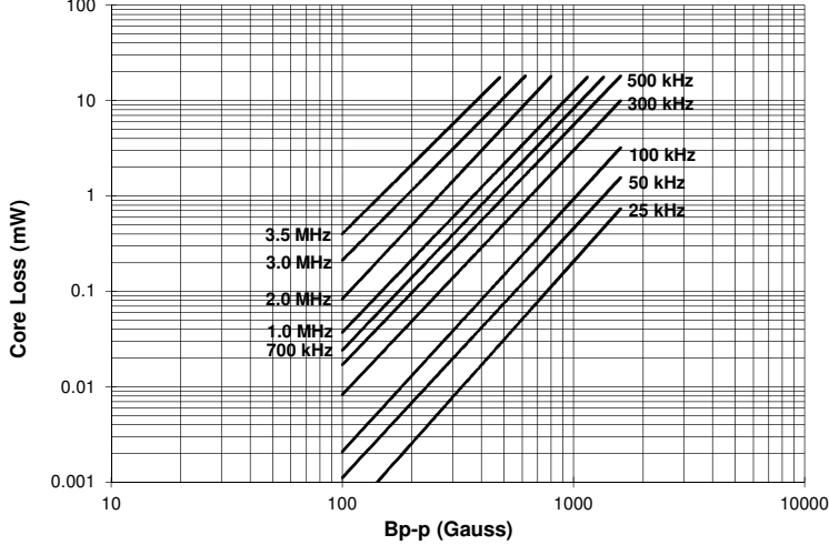
MPIA4012V2-1R5-R
