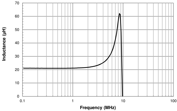
MPIA4020V2-220-R
