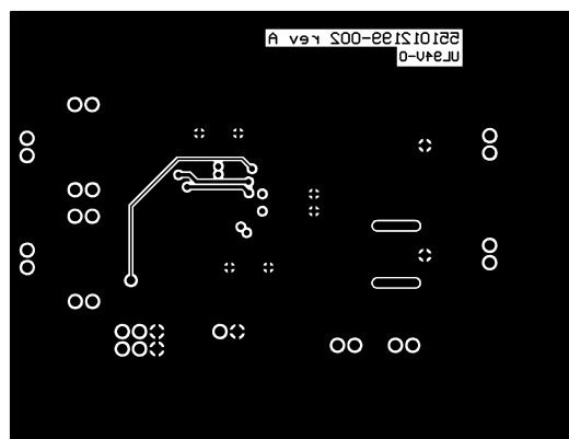
Bottom Layer
