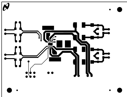
Top Layer
