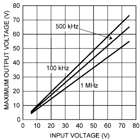
V_{O-MAX} vs V_{IN} , LM3406
