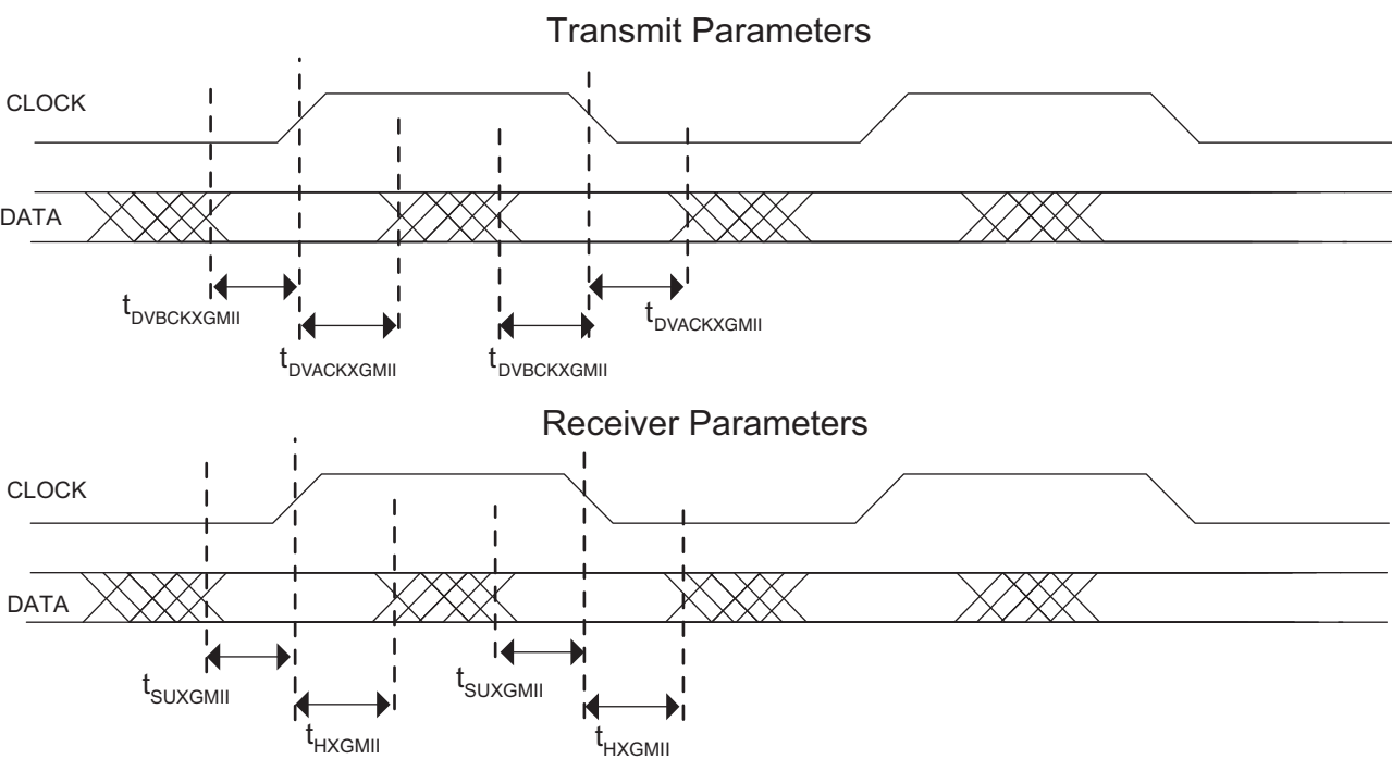
Figure 3-8. XGMII Parameters
