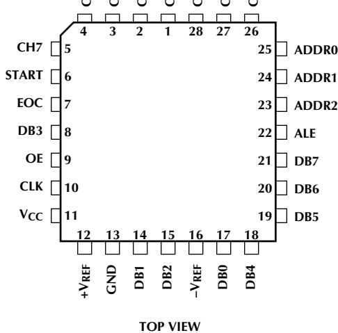
ML2259 28-Pin PLCC (Q28)
