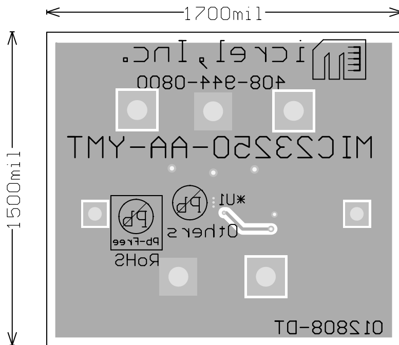
Bottom Layer
