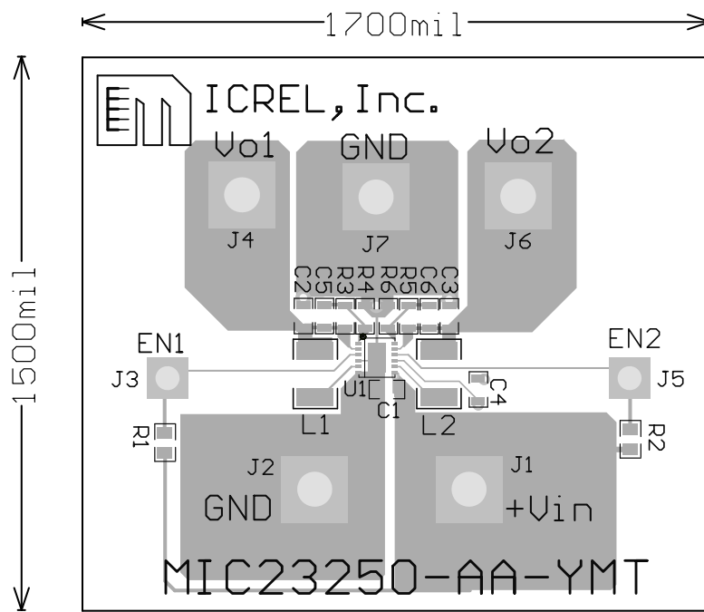
Top Layer
