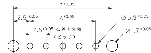
基板取付穴推奨寸法 ( t = 1.6 \pm 0.05 )
