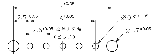
基板取付穴推奨寸法
