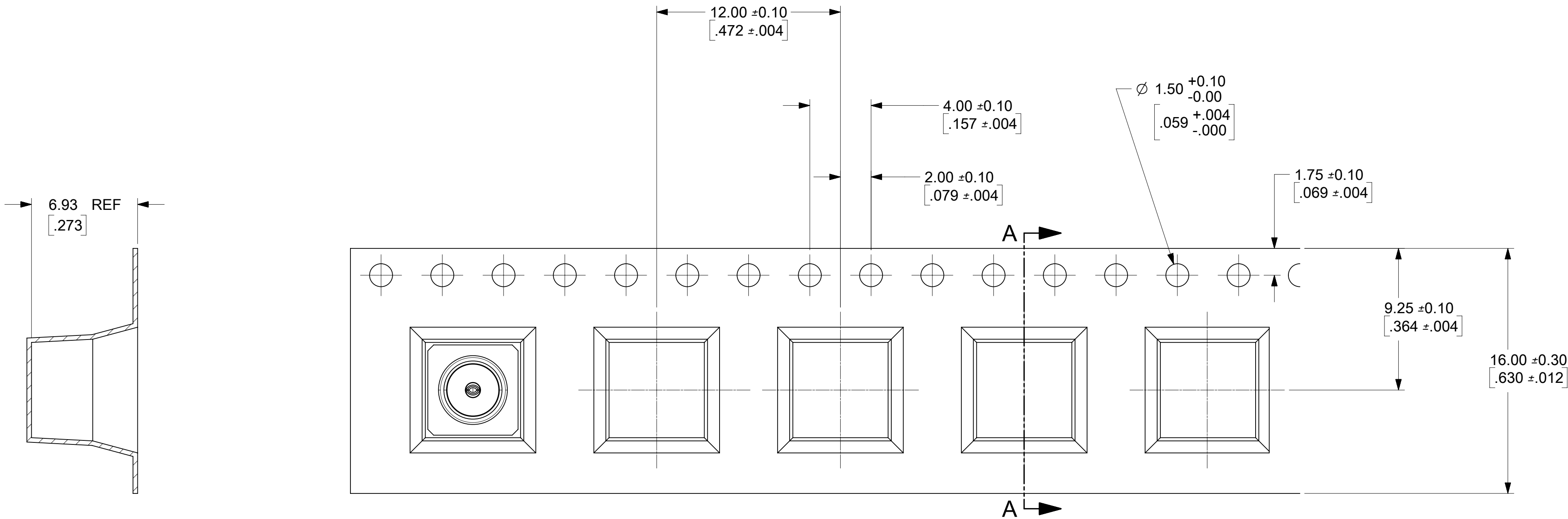
SECTION A-A
