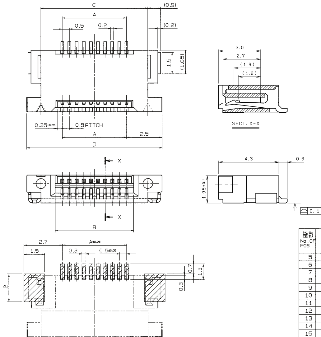
推奨基板取付け寸法 (コネクタ搭載側)
