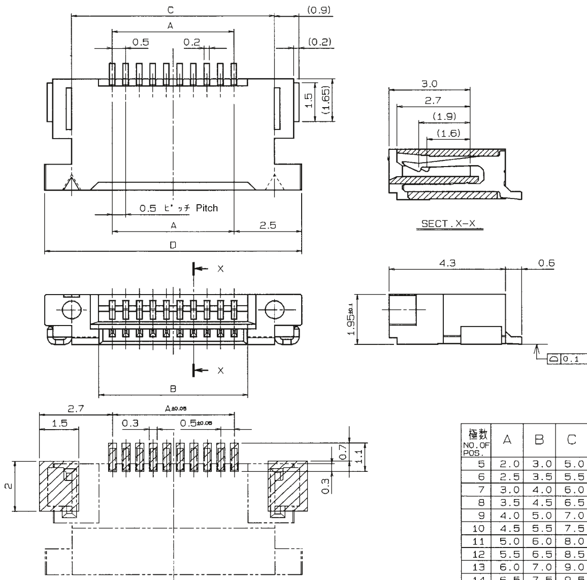
推奨基板取付け寸法 (コネクタ搭載側) MOUNTING LAYOUT (CONN. MOUNTING SIDE)
