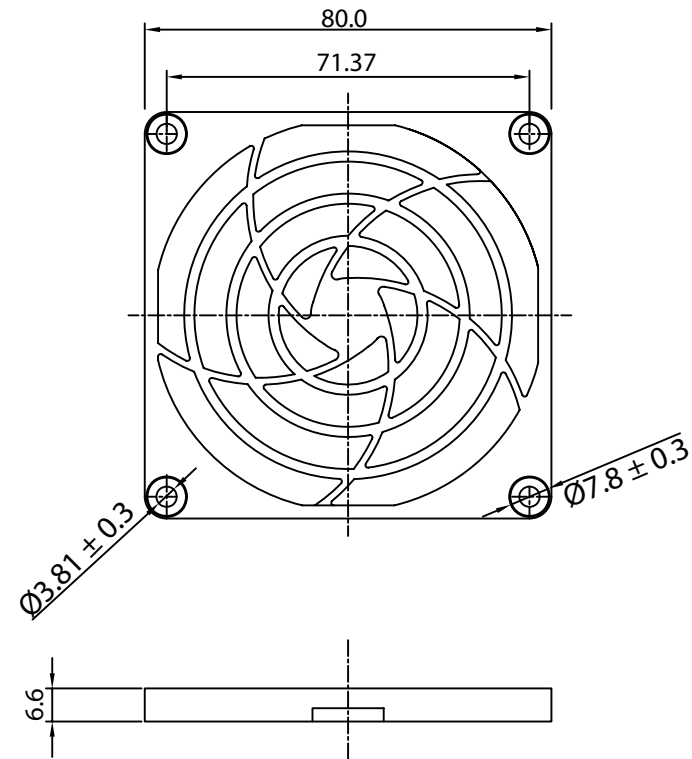
FAN GUARD
