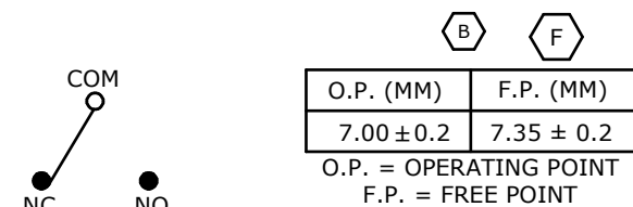
CIRCUIT: SPDT
