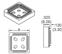
图 1 - 通孔安装
