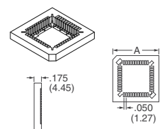
图 2 - 表面贴装
