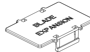
10042774-002 10042774-002LF 10042774-003 10042774-003LF SCALE 1:1
