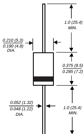
DO-201AD
