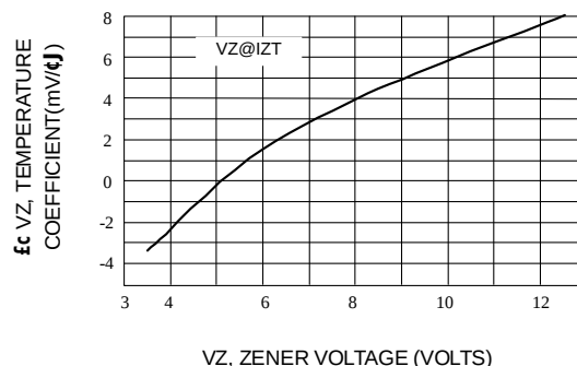
Fig. 2-ZENER VOLTAGE-TO 12 VOLTS
