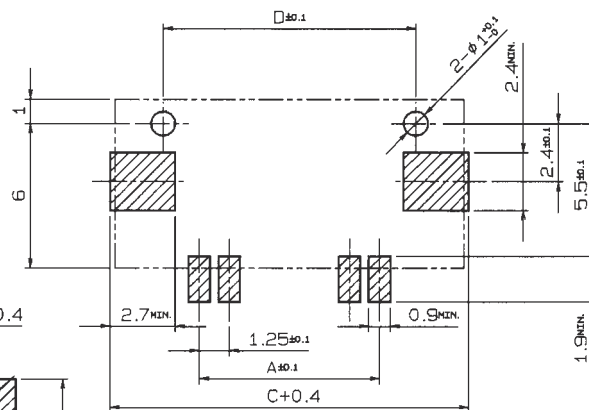
基板取付け寸法コネクタ搭載側より見た図
