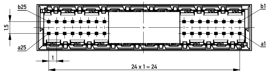
Leiterplatten-Layout Vorschlag / PCB-layout proposal
