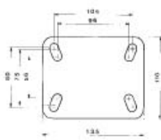
Ø 80-100/50-160/50
