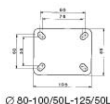
Ø 80-100/50L-125/50L
