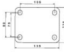
Ø 125/60-250/60
