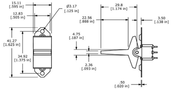
R16 Actuator
