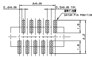
基板取付け寸法 (コネクタ搭載面側) MOUNTING LAYOUT (CONN. MOUNTING SIDE)
