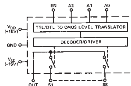
AD7501/AD7503
