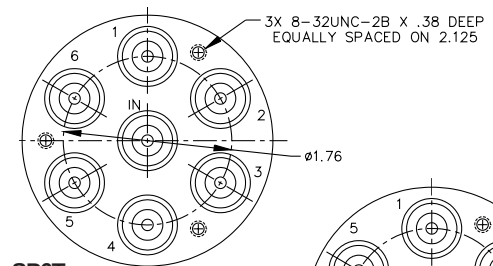
SP6T
