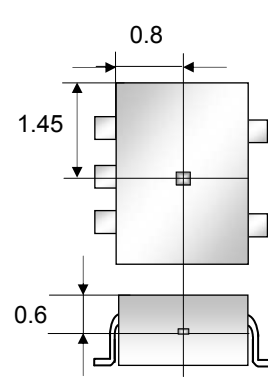
SSOP5
