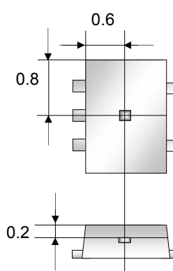
HVSO5
