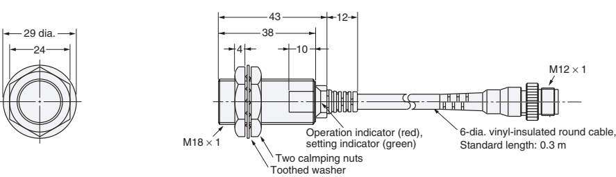
Fig. 31 : E2E-X7D1-M1GJ E2E-X7D1-M1J-T
