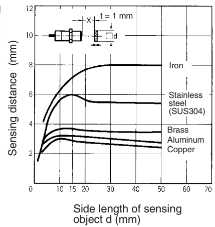
E2E-X1R5E / F E2E-X1R5Y
