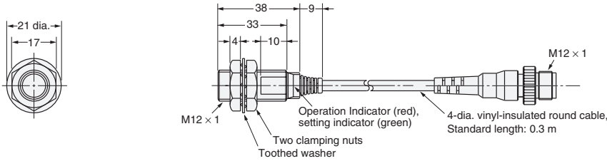
Fig. 29 : E2E-X3D1-M1GJ E2E-X3D1-M1J-T
