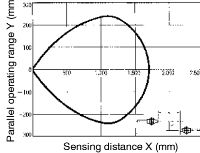
E32-T11L with E3X-NH amplifier
