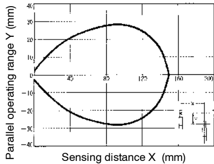
E32-T24 with E3X-NH amplifier
