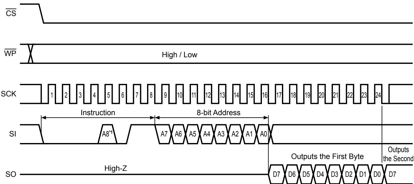
图 16 READ 工作 (S-25A010A/020A)
