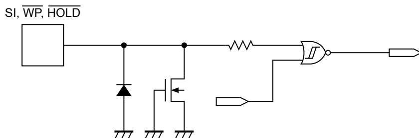
图 25 SI, \overline{WP} , \overline{HOLD} 端子
