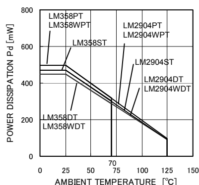
LM358DR/PWR/DGKR LM2904DR/PWR/DGKR/VQDR/VQPWR
