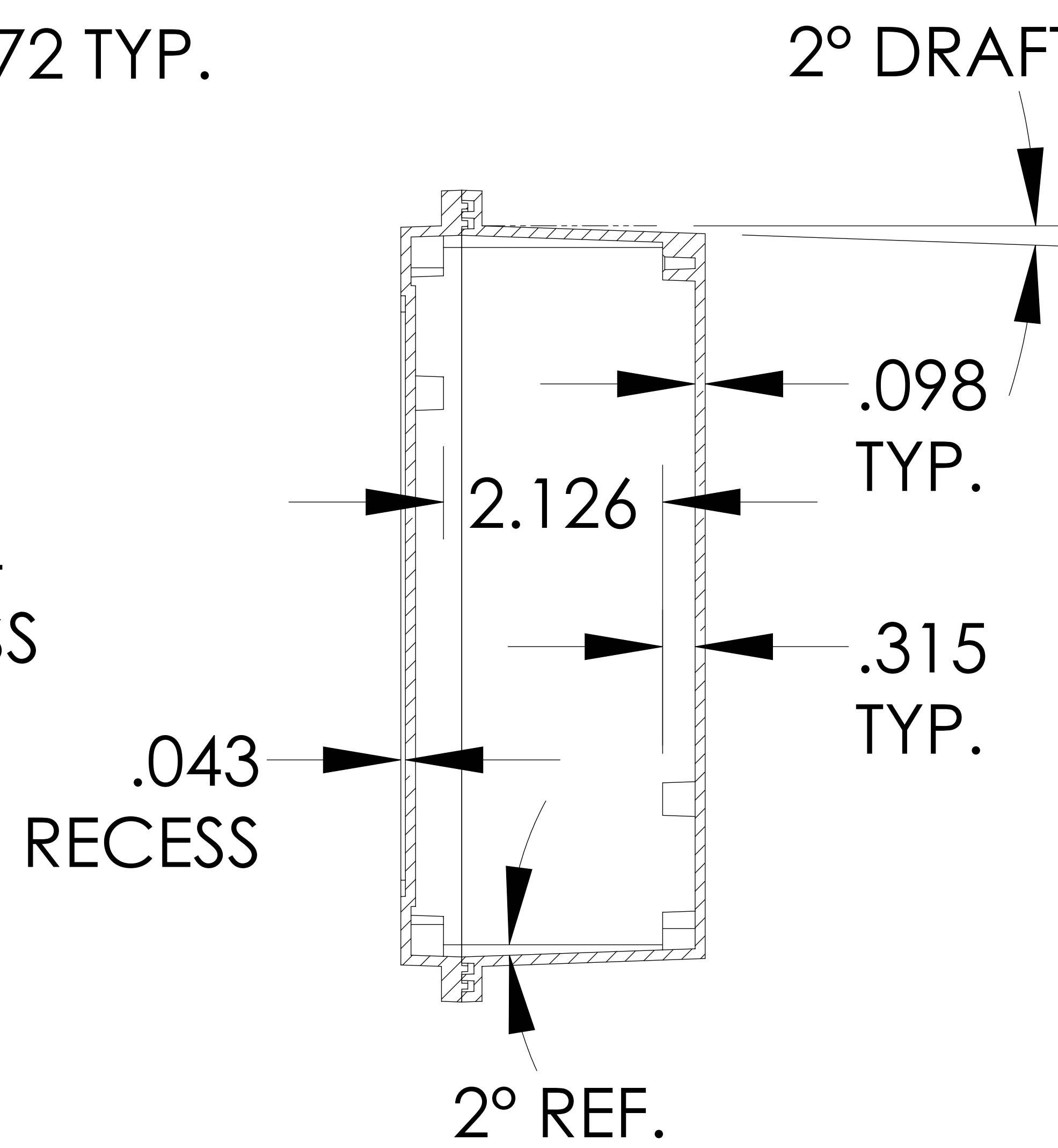
SECTION A-A
