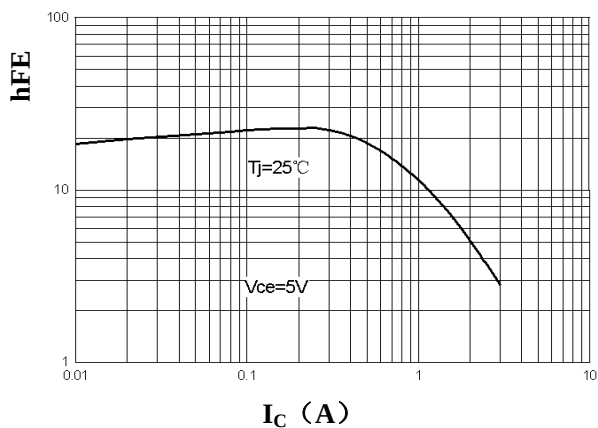
h_{FE} - I_C
