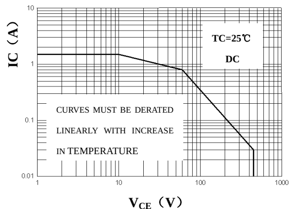
SOA
