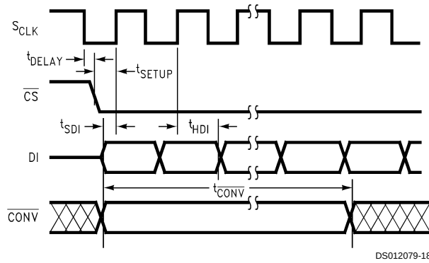
DI Data Input Timing
