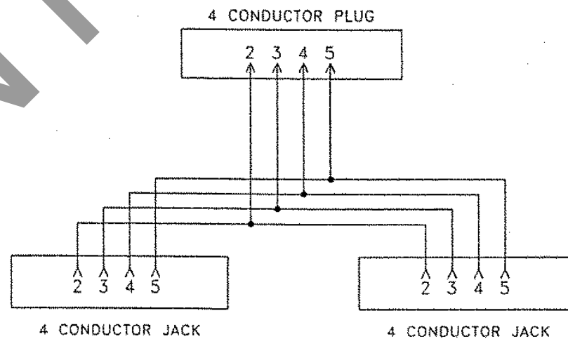
WIRING SCHEMATIC
