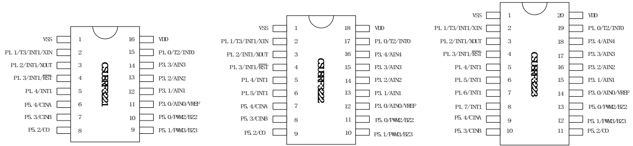
图1 16/18/20-pin 配置图
