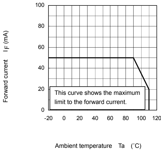
I_F - T_a
