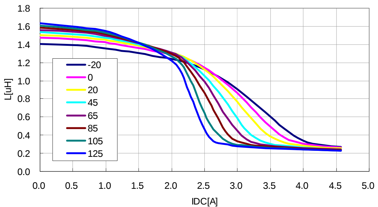
VLS3012T-1R5N1R7
