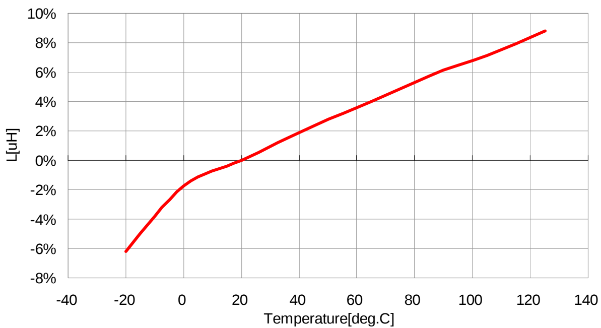
VLS3012T-1R5N1R7
