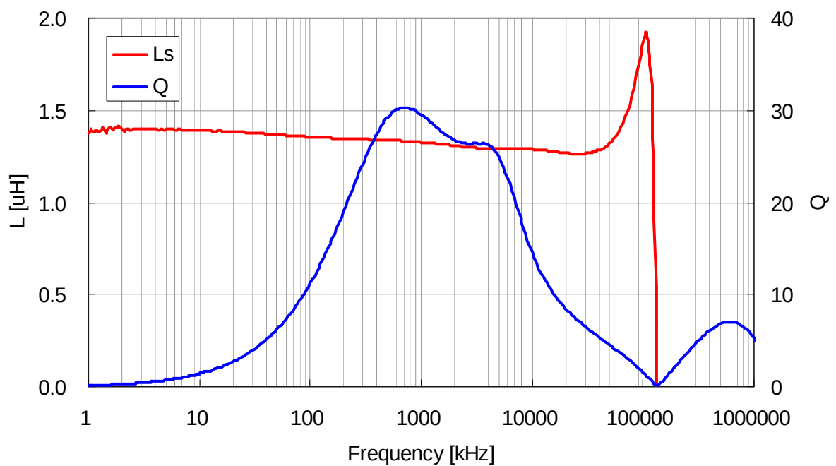
VLS3012T-1R5N1R7
