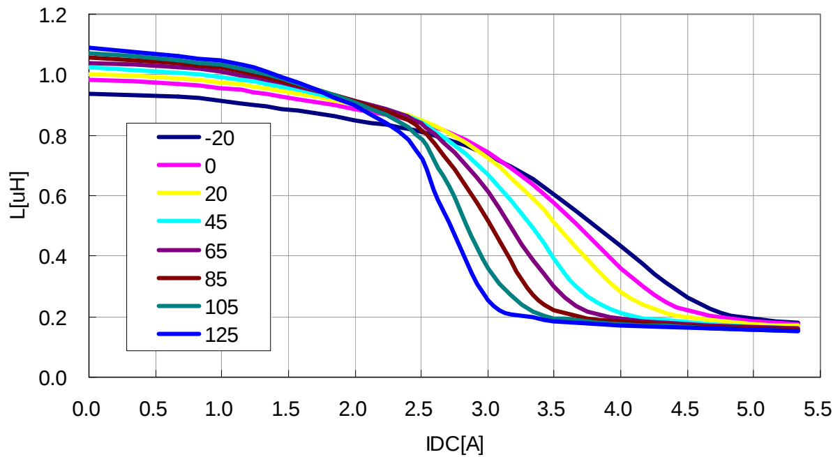
VLS3012T-1R0N2R2
