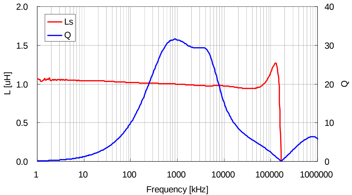
VLS3012T-1R0N2R2
