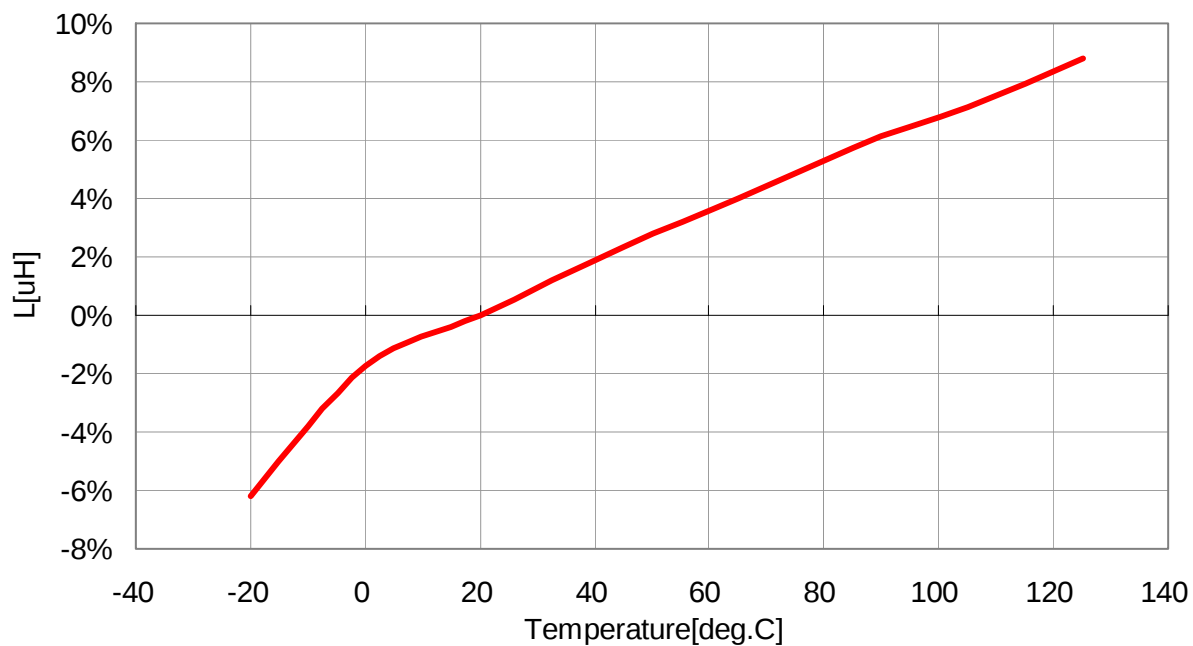
VLS3012T-1R0N2R2
