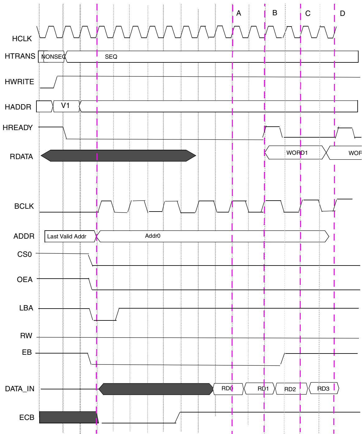
Figure 62. FCE=0,SYNC=1,BCD=1,WSC=8,BCS=0,CSA=0,OEA=0
