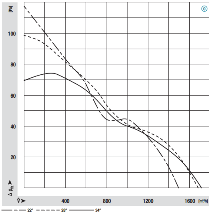
M4Q045-EF01-**, Ø 300, 50 Hz
