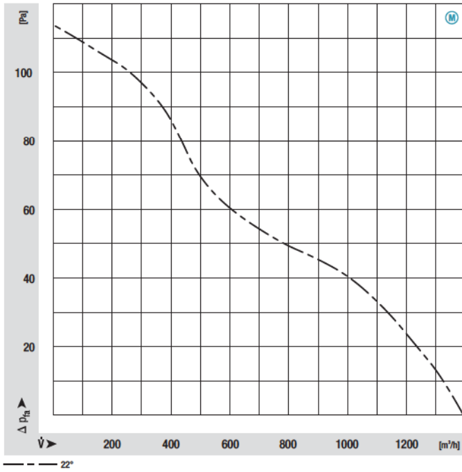
M4Q045-EA01-**, Ø 300, 50 Hz
