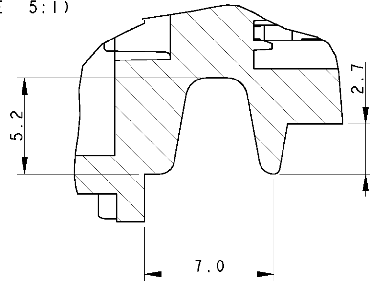
DETTAGLIO H SCALA 5:1 (DETAIL H SCALE 5:1)
