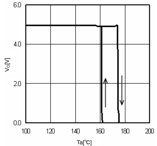
Fig.16 TSD ( I_O=0mA )
