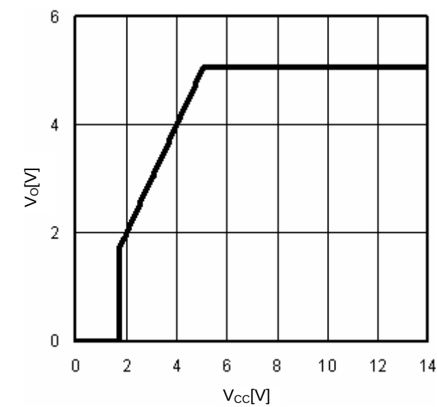
Fig.15 V_{CC}-V_O ( I_O=0mA )
