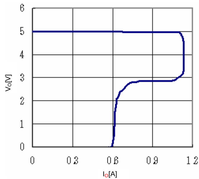
Fig.17 OCP
