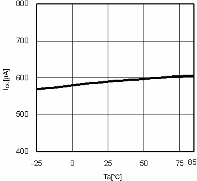
Fig.10 Ta-I CC
